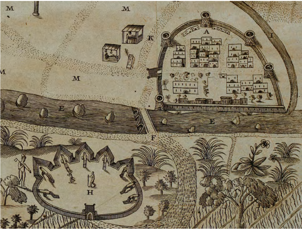
Jean-Baptiste Tavernier, 1679
